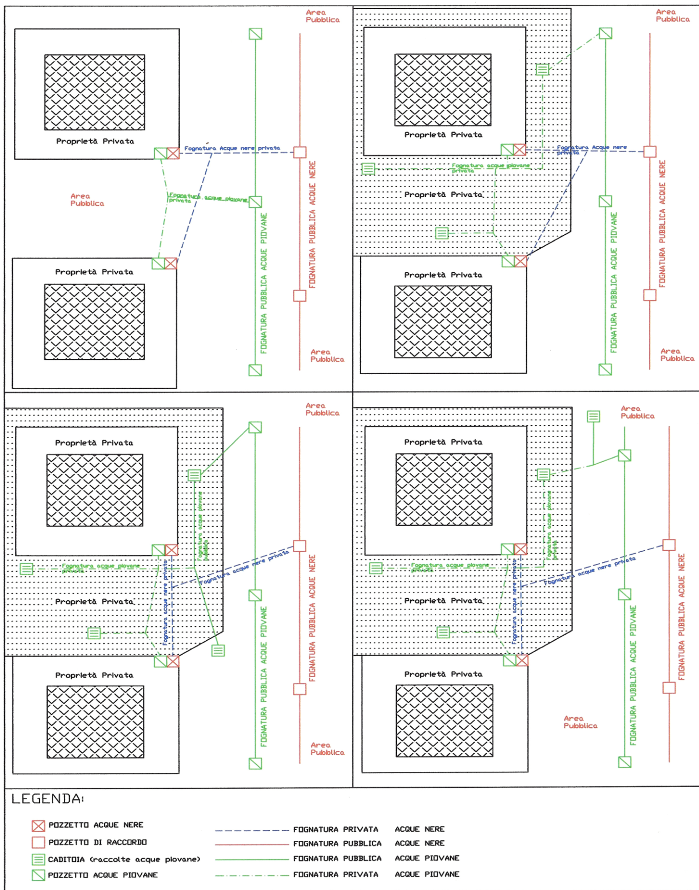
Fig. 1.b: Esempi esplicativi per la definizione di fognatura privata in caso di fognatura pubblica separata
