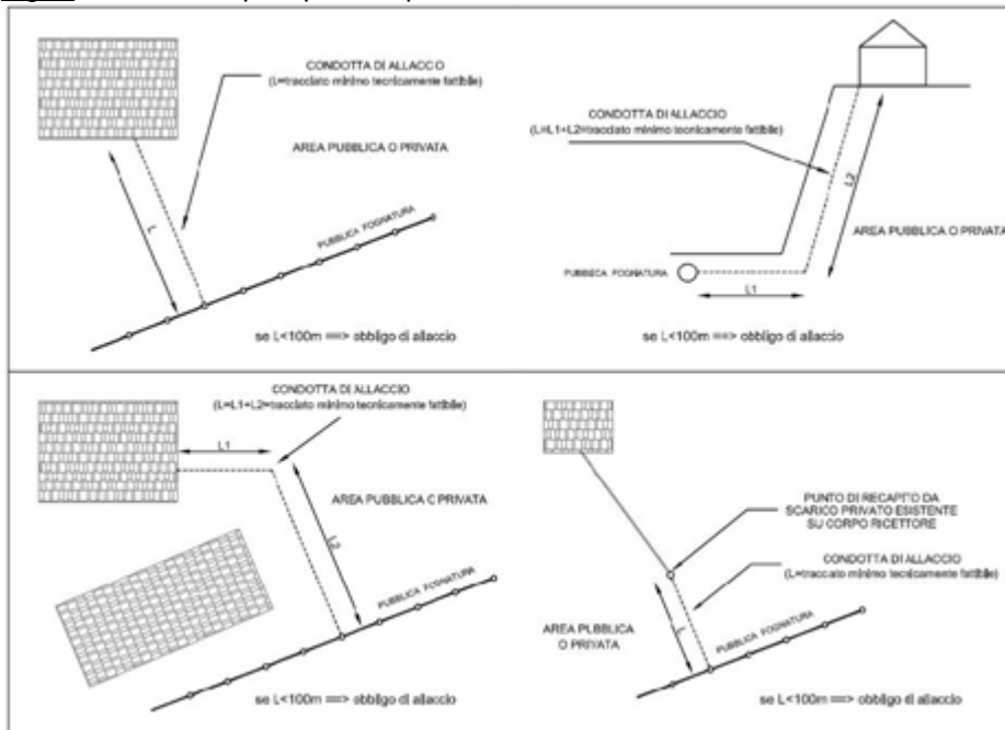
Fig. 3: alcuni esempi esplicativi per la definizione tracciato tecnicamente fattibile
