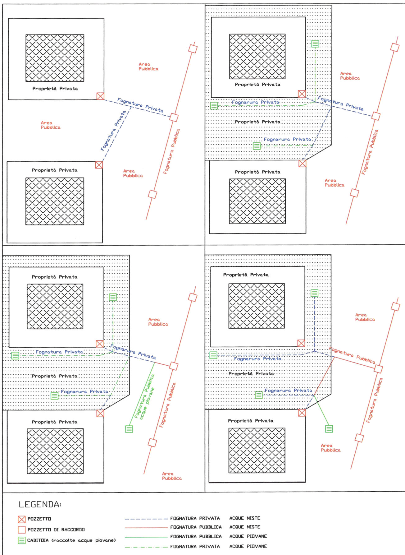
Fig. 1.a: Esempi esplicativi per la definizione di fognatura privata in caso di fognatura pubblica mista.
